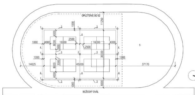
PÓDORYS KURTU PRE PLÁŽOVÝ VOLEJBAL M 1:500
